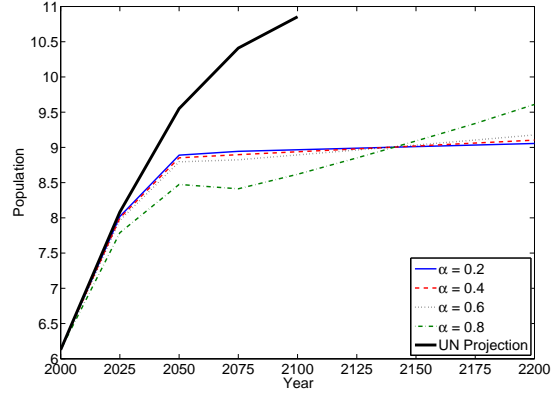
(d) \hat{\beta} = 0.9925
