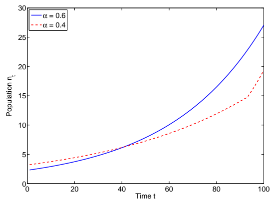
(d) \eta = 0.015
