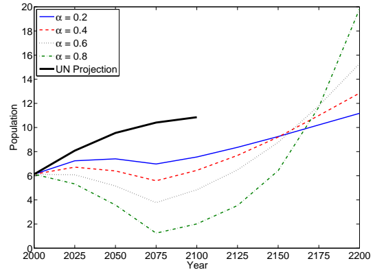
(d) \hat{\beta} = 0.9925
