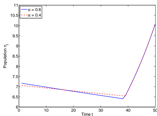
(d) \eta = 0.015
