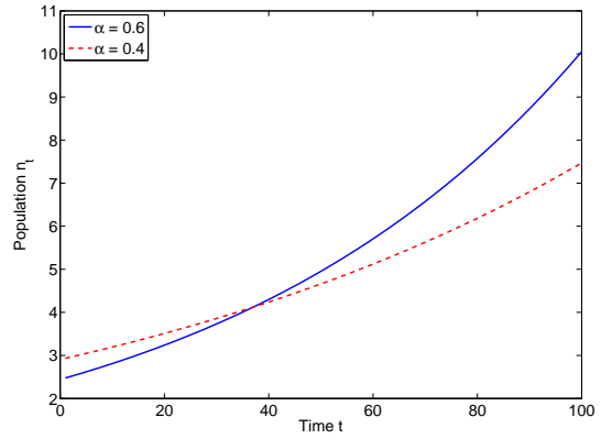
(d) \beta = 0.975
